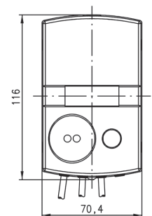
Vorderansicht Rechenwerk
